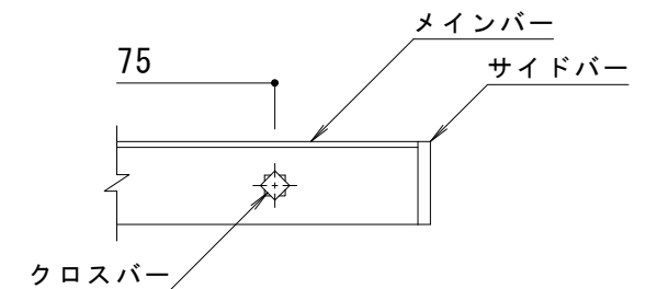
C-C断面図
