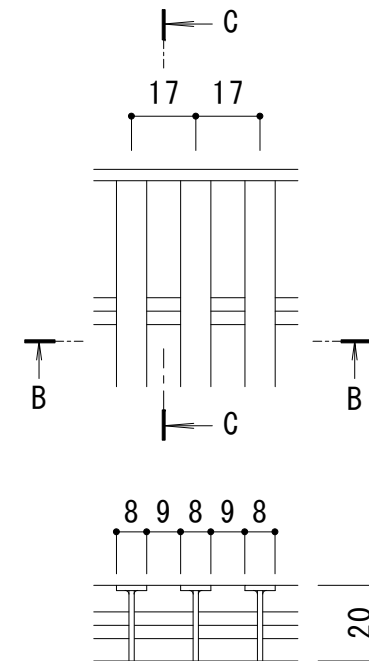
B-B断面図
