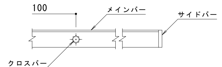
C-C断面図
