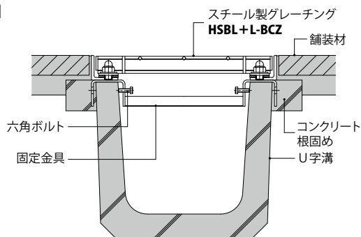
納まり図
