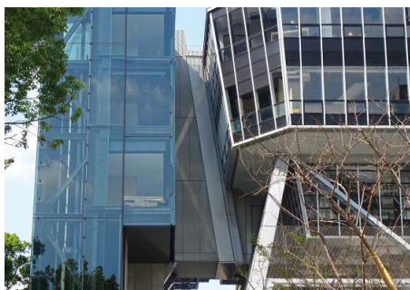
免震エキスパンションジョイント 外壁部 斜めクリアランス対応仕様
