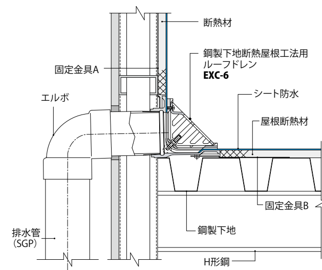
EXC-6-100 納まり図
