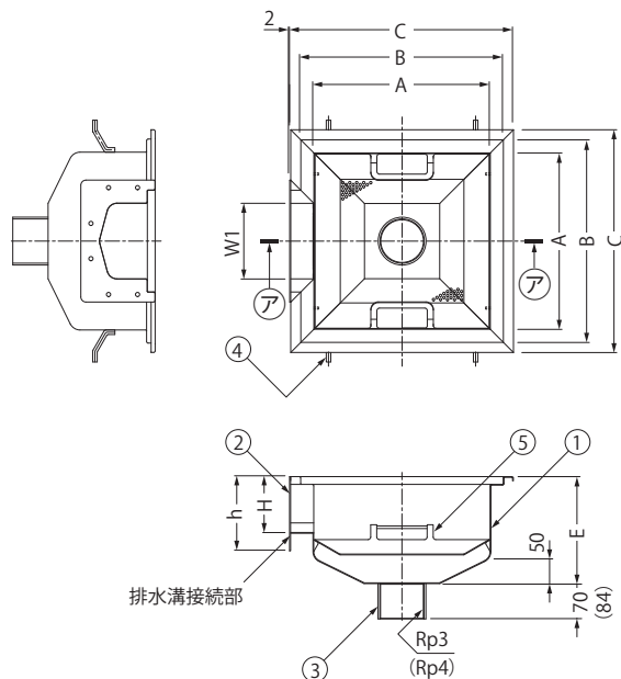
⑦-⑦断面図
