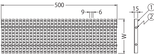
集水樹蓋
