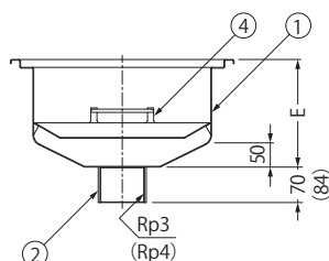
ア-ア断面図
