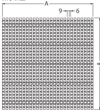
集水樹蓋
