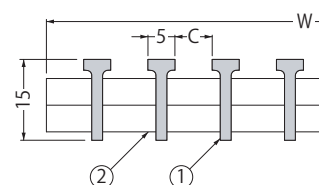
断面詳細図
