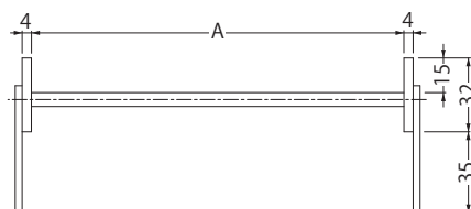
断面詳細図
