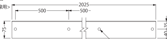
<曲線用>
