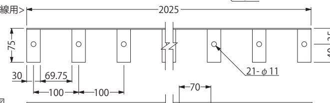
<曲線用>
