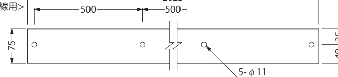
<曲線用>
