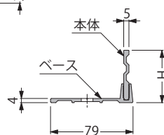
A-A断面図
