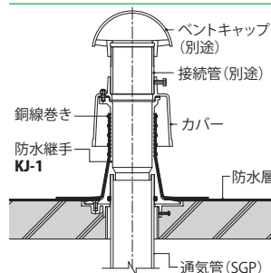
KJ-1 納まり図
