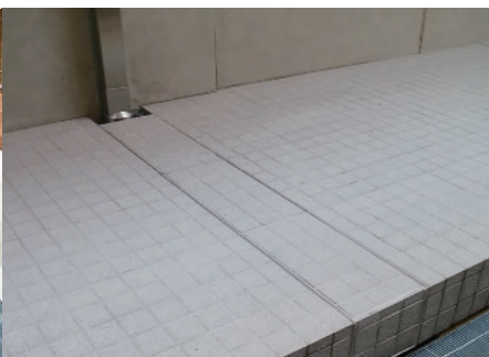
屋外床部 免震エキスパンションジョイント 曲線クリアランス対応仕様
