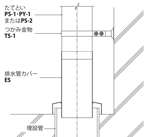
排水管カバーES・たてといPY-1
