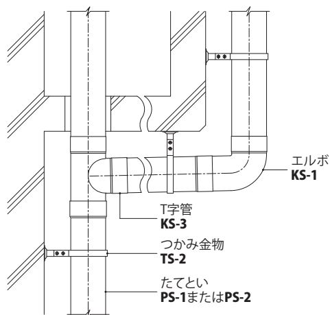
エルボKS-1・KS-3・つかみ金物TS-2
