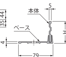
A-A断面図
