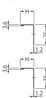
断面図
