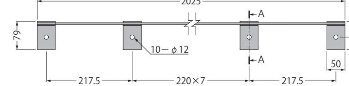
背面図
