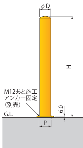
寸法・質量表
