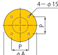
ベースプレート寸法表
