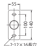
ベースプレート詳細
