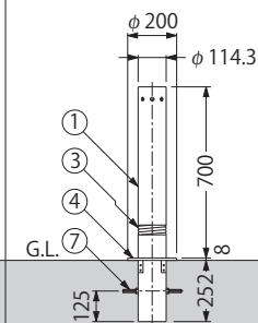
チェーン内蔵タイプ UK1170SC (受注生産品) チェーン端部用 UK1170SE (受注生産品) チェーンなし UK1170SN (受注生産品)
