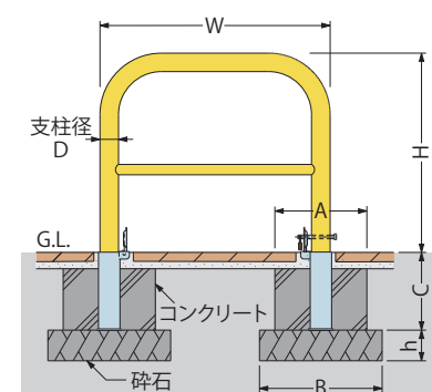
アーチ型 納まり図
