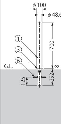
チェーン内蔵タイプ UK0470C (受注生産品) チェーン端部用 UK0470E (受注生産品) チェーンなし UK0470N (受注生産品)
