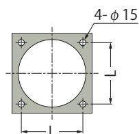
フックボルト取付寸法
